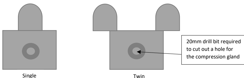
Fig 3 End cap
